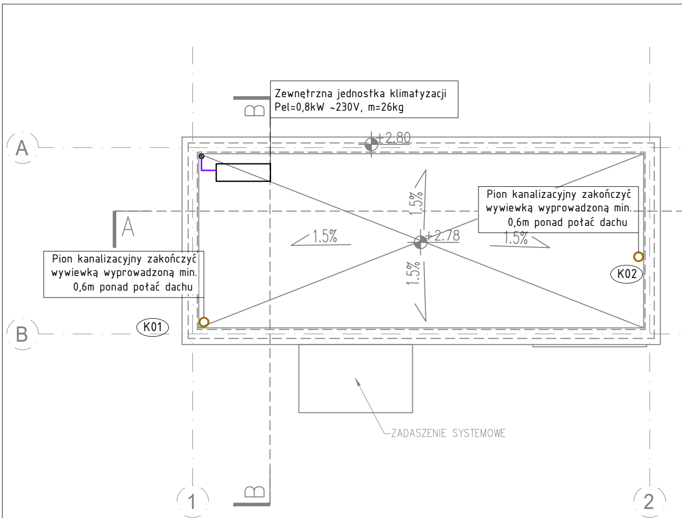
RZUT DACHU
